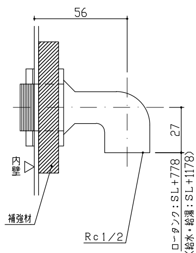
給水・給湯・ロータンク給水接続
