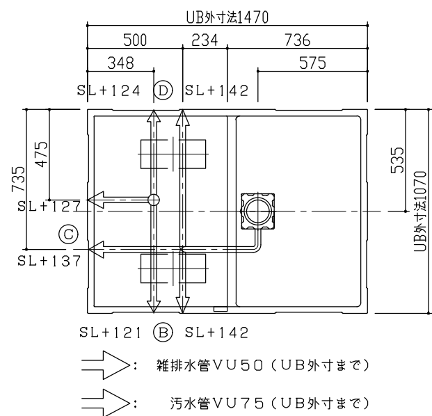
雑排水取出し可能方向 S=1/20
