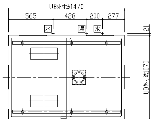
給水・給湯取出し位置 S=1/20
