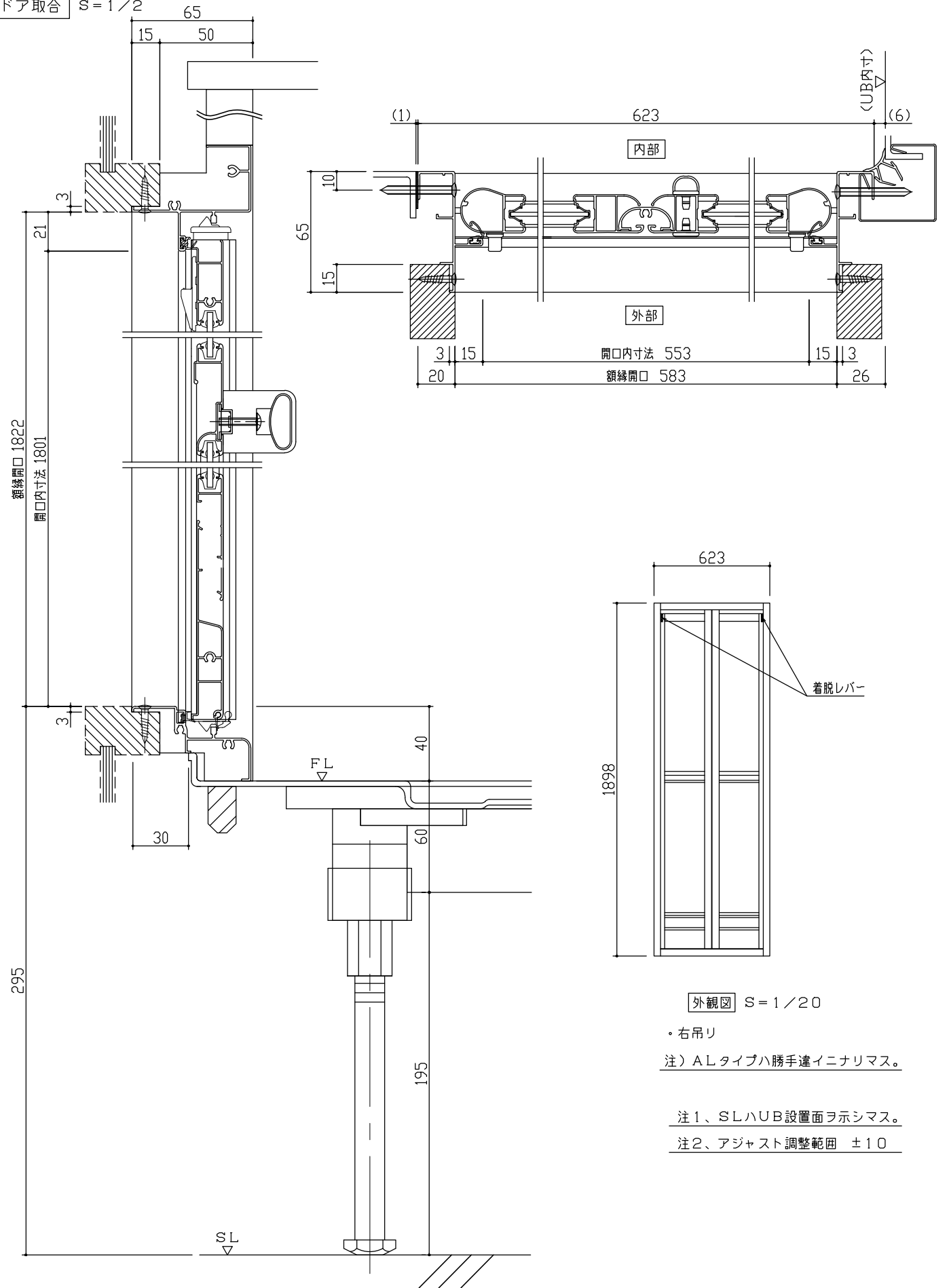
ドア取合 S=1/2
