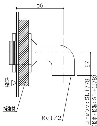
給水・給湯・ロータンク給水接続
