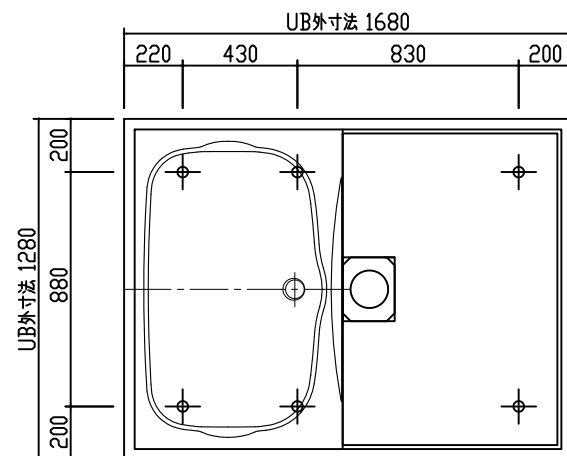
脚位置図 S=1/20
