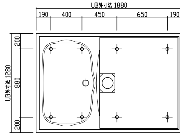
脚位置図 S=1/20
