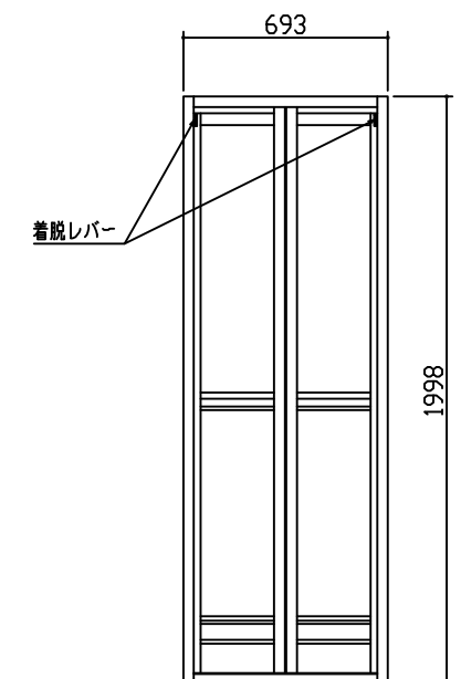
外觀図 S = 1 / 20
