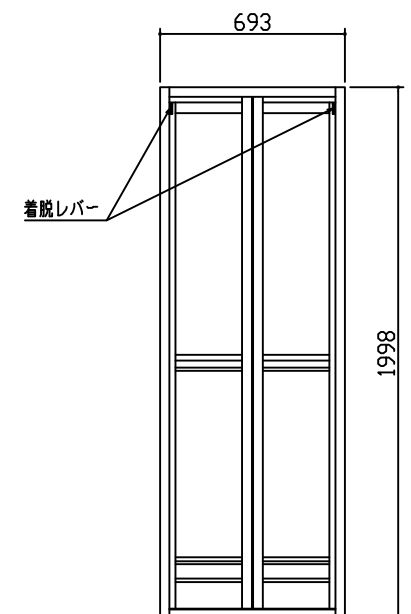
外觀図 S = 1 / 20
