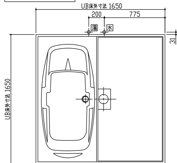
雑排水取出し可能方向 S = 1 / 20
