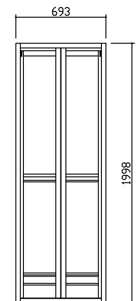
外觀図 S=1/20
