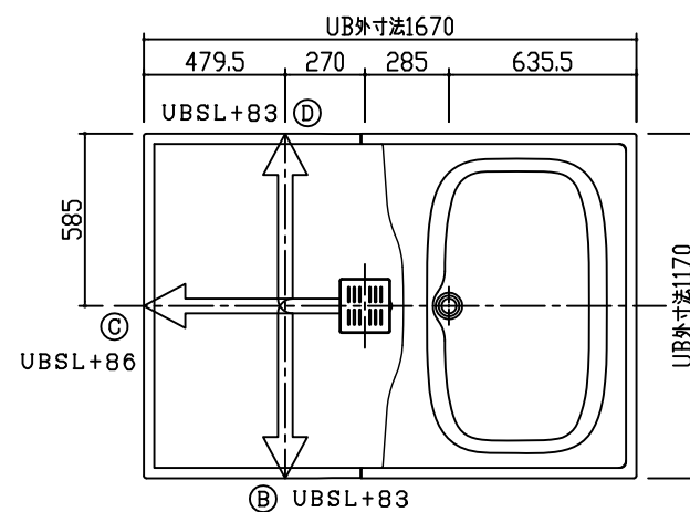
雑排水取り出し可能方向 S=1/20
