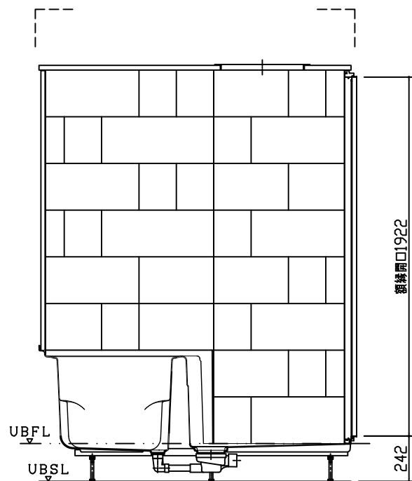
B 面
