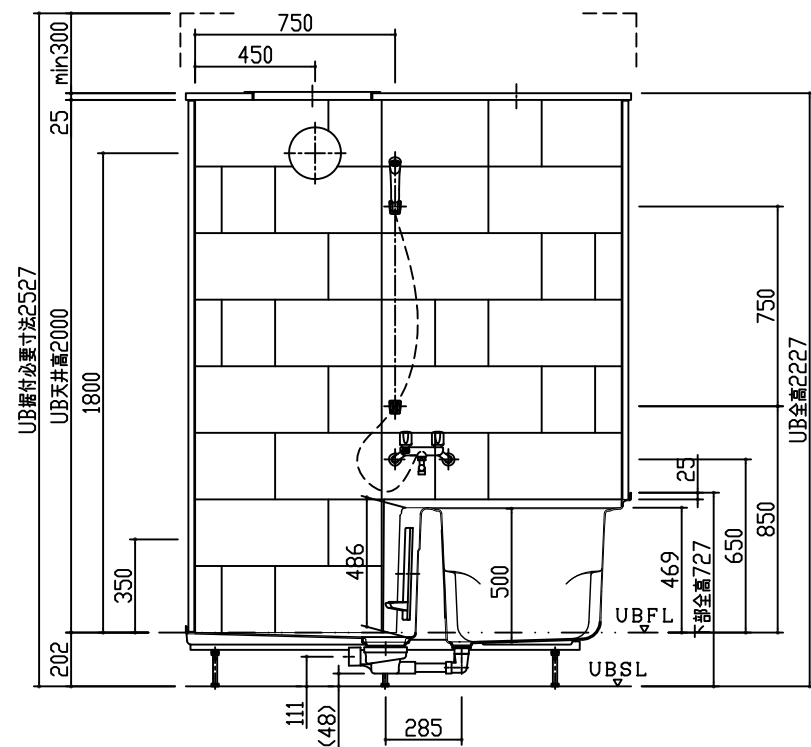
D 面
