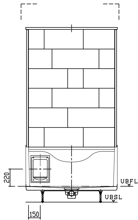
A 面
