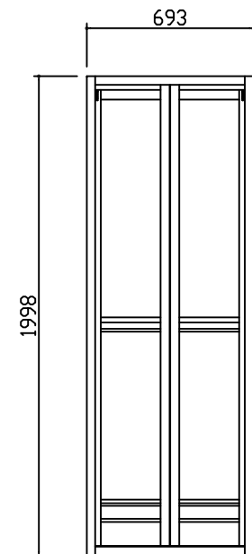
外観図 S=1/20
