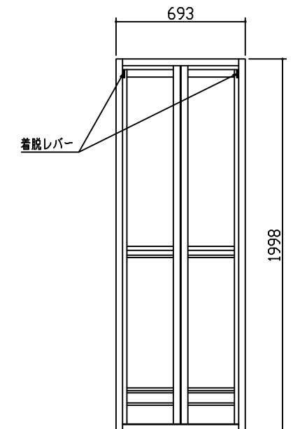
外観図 S=1/20
