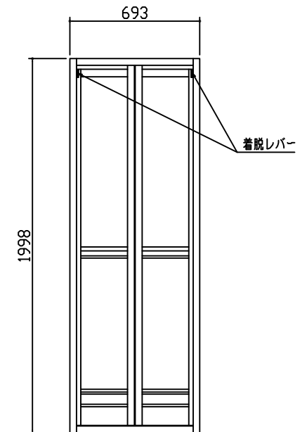
外観図 S=1/20
