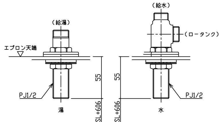
給水・給湯・ロータンク給水接続
