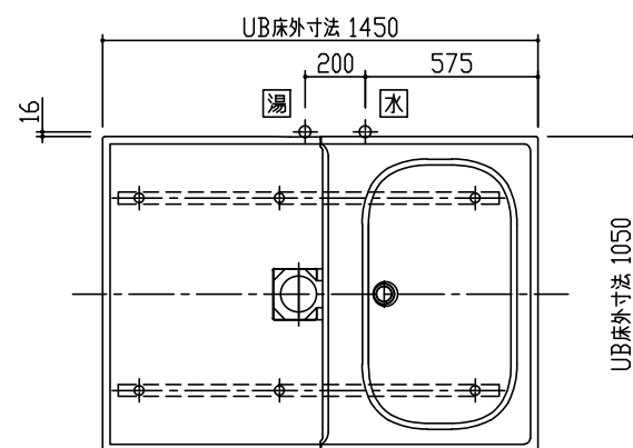
給水・給湯取出し位置 S=1/20
