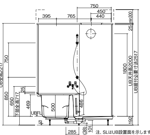
● 立面図
