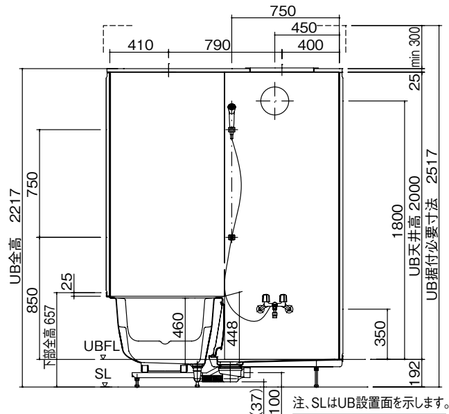
●立面図
