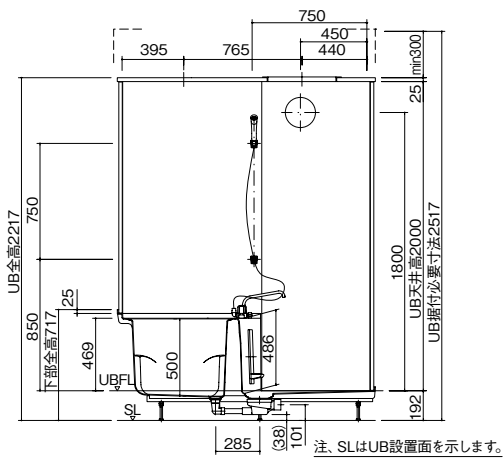
● 立面図
