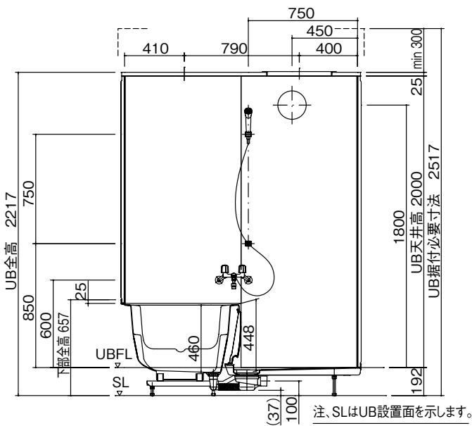
●立面図
