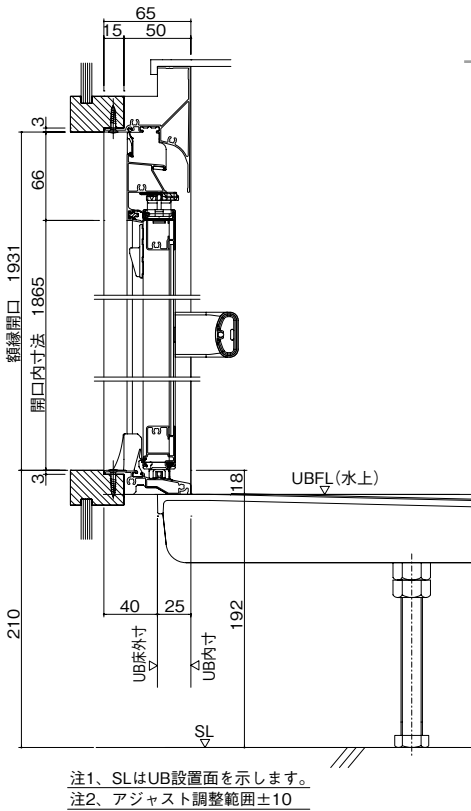
●ドア取り合い
