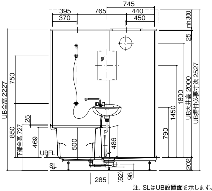
●立面図
