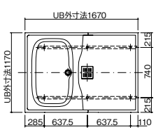
● 脚位置図
