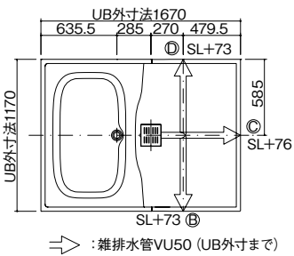
●雑排水 取出し可能方向
