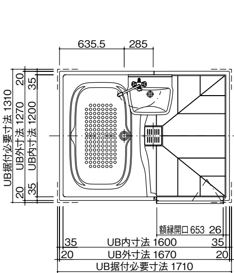
●平面図
