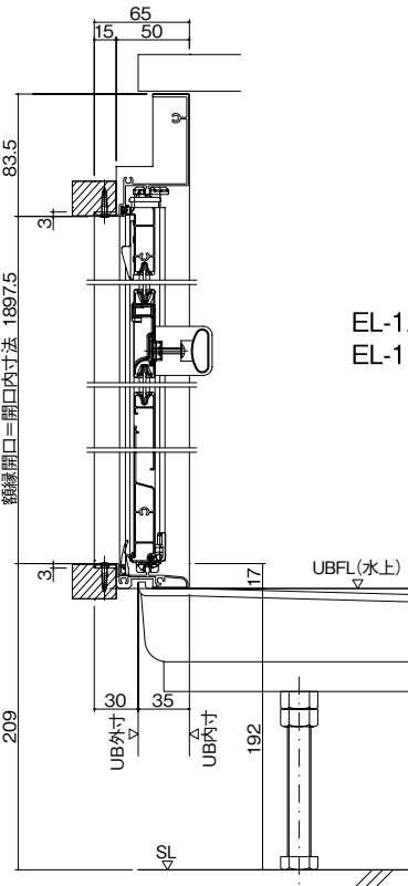
●ドア取り合い
