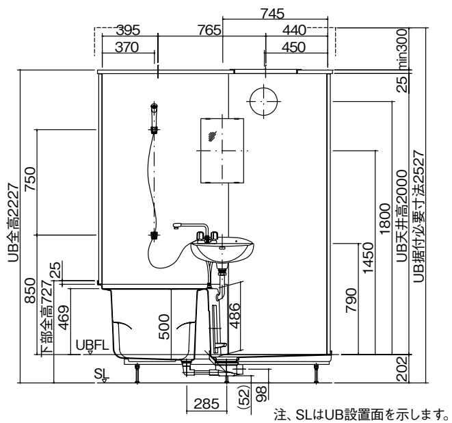
●立面図
