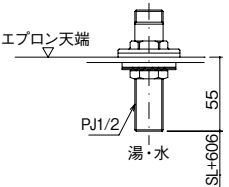
●給水・給湯 接続部
