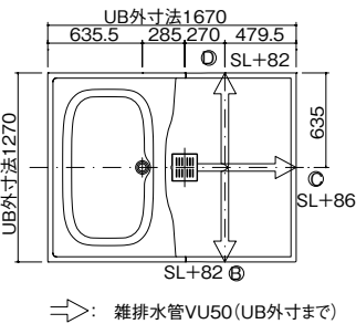
●雑排水 取出し可能方向
