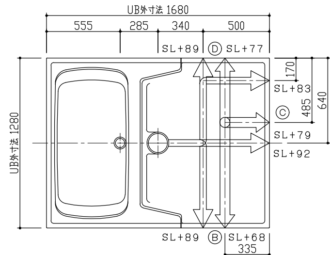
雑排水取出し可能方向 S=1/20
