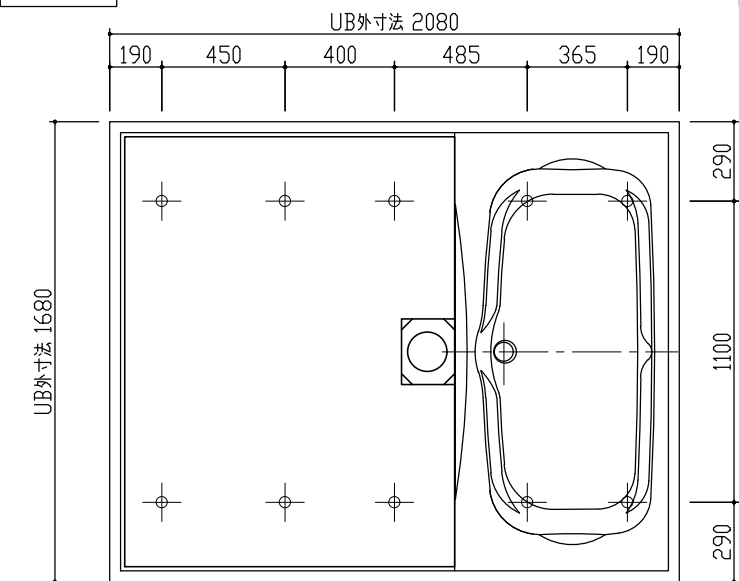
給水・給湯取出し位置 S = 1 / 20
