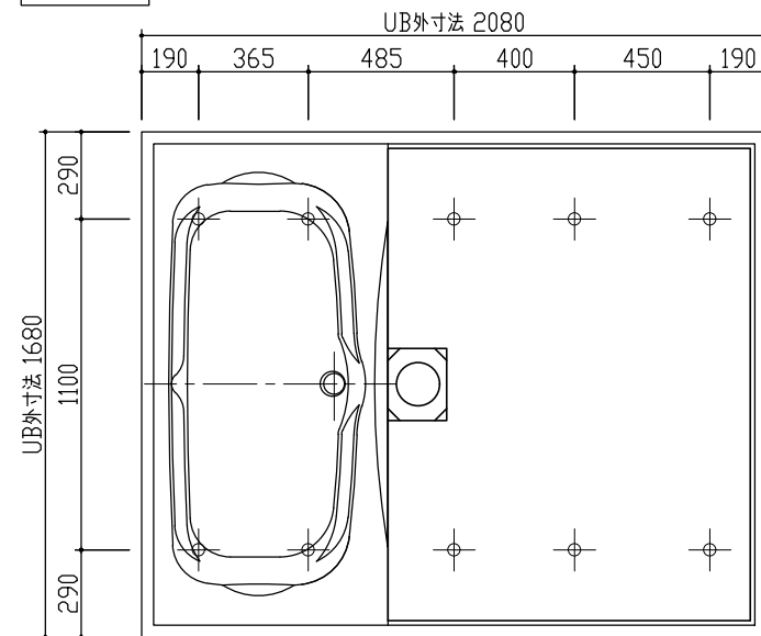
給水・給湯取だし位置 S=1/20
