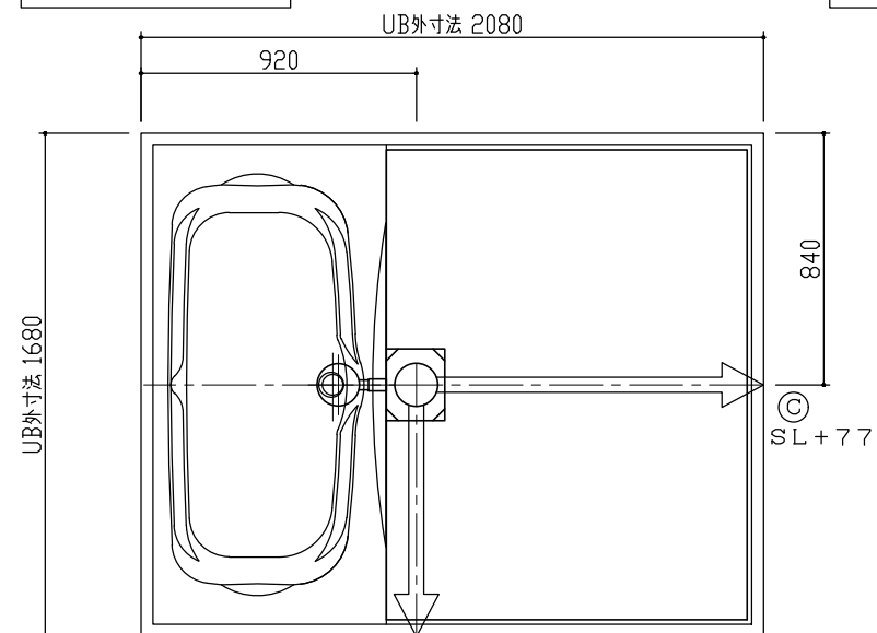
雑排水取り出し可能方向 S = 1 / 20
