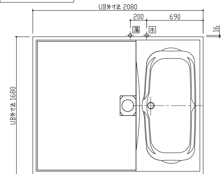
雑排水取出し可能方向 S = 1 / 20
