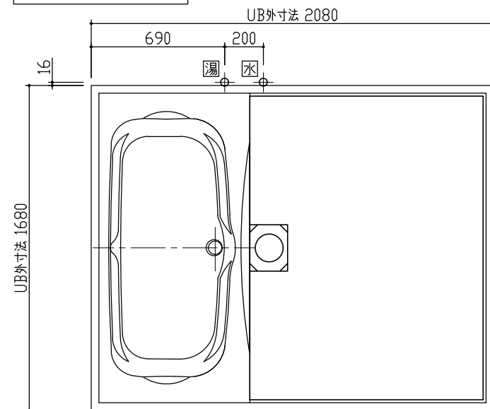
雑排水取り出し可能方向 S = 1 / 20
