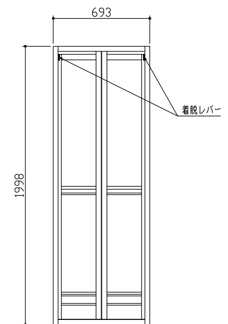
外觀図 S = 1 / 20
